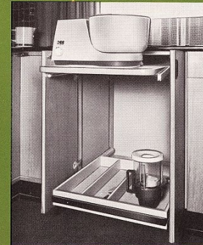
Type OU med dobbeltåbning. Mont. med kraftig specialbeslag til røremaskine. Alle fremtræksbeslag er låst i arbejdsstillingen. Forednen i skabet kan indsættes i kassette eller trådkurve efter ønske og behov.
