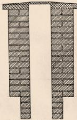
Snit D-E.
